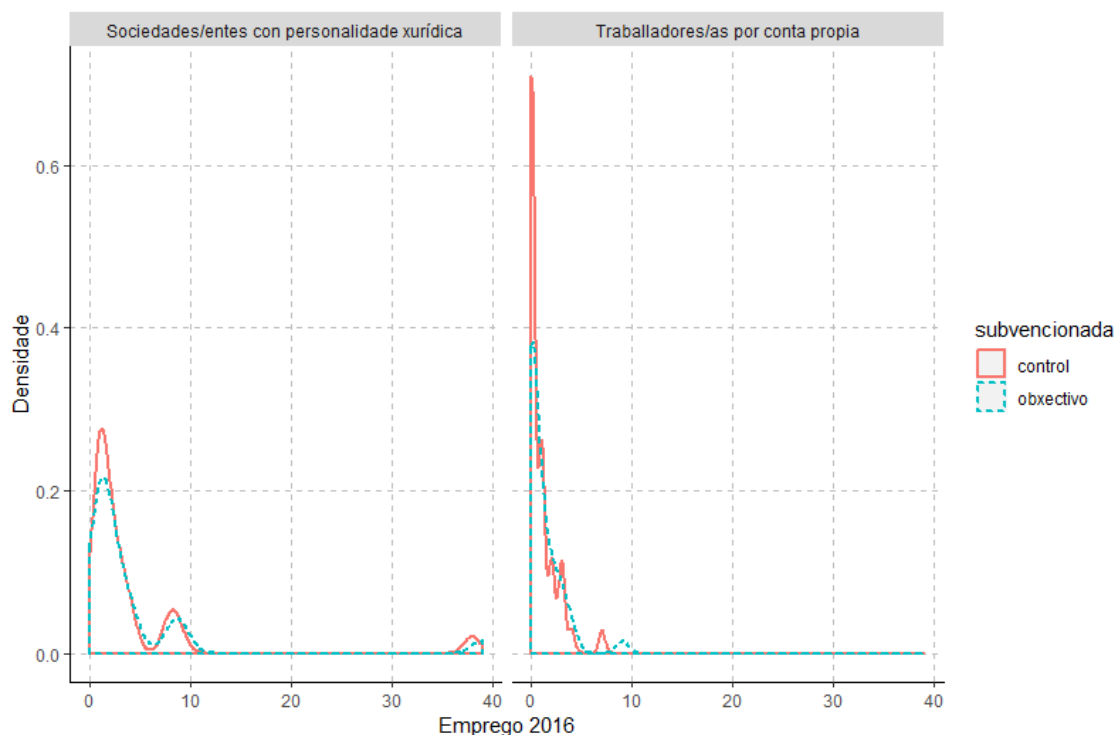
Gráfico 4. Funciones de densidad del empleo en 2016 de las empresas objetivo y control según el tipo de empresa
