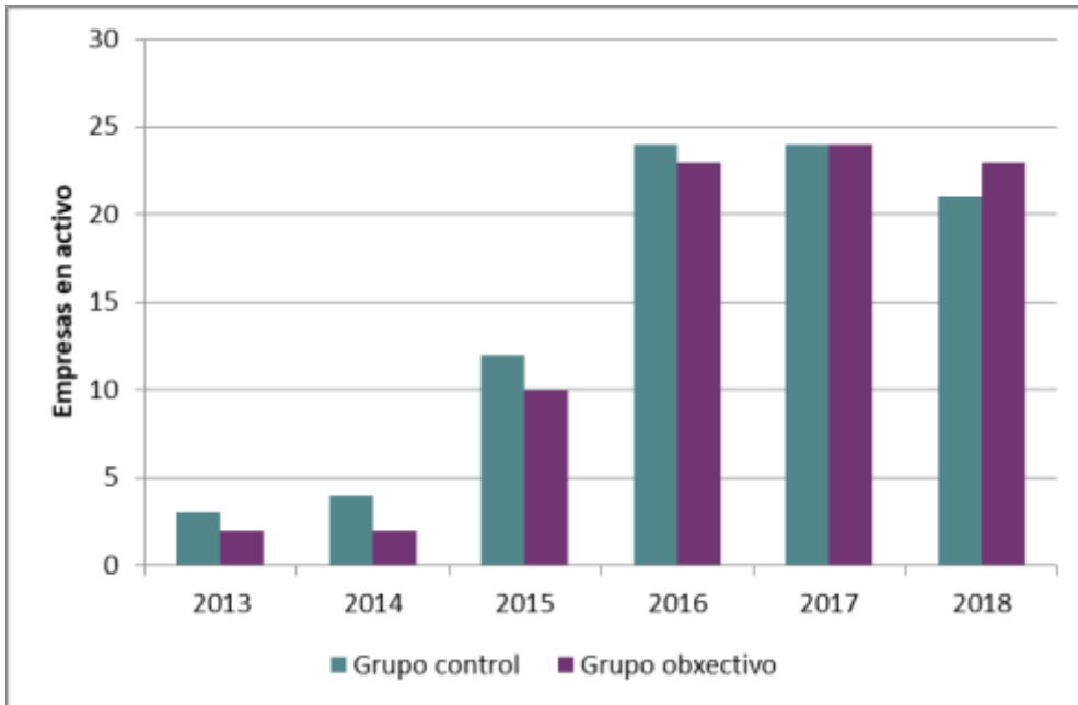
Gráfico 12. Comparativa de la supervivencia (empresas que continúan en activo en Galicia) de los grupos subvencionado (objetivo) y no subvencionado (control) para el grupo de sociedades/entes con personalidad jurídica
