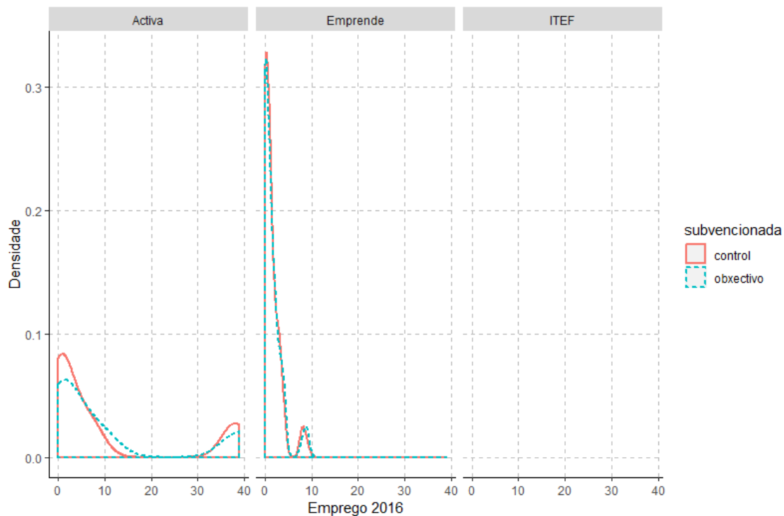
Gráfico 5. Funciones de densidad del empleo en 2016 de las empresas objetivo y control agrupándolas en base a la línea de ayuda recibida
