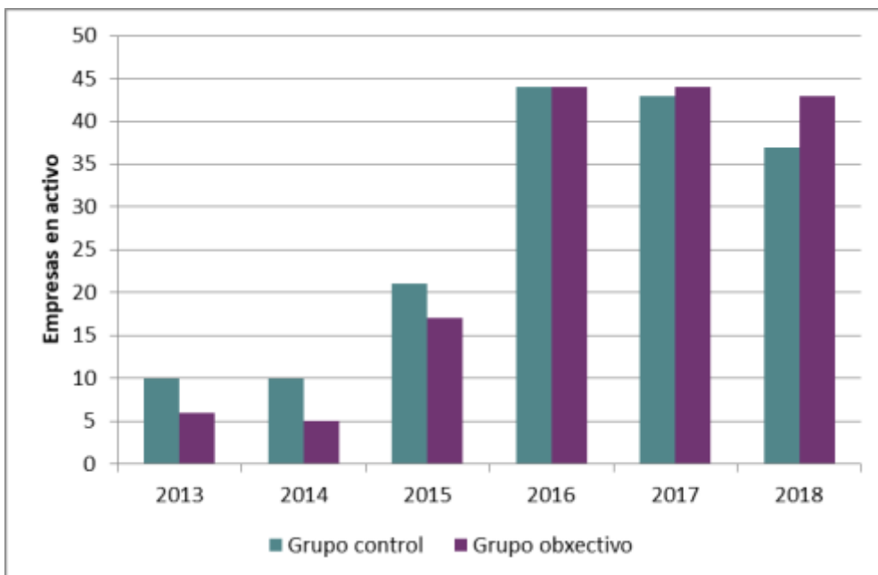
Gráfico 13. Comparativa de la supervivencia (empresas que continúan en activo en Galicia) de los grupos subvencionado (objetivo) y no subvencionado (control) para el grupo de trabajadores/as por cuenta propia
