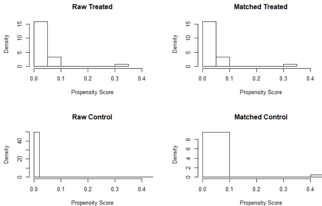
Gráfico 1. Histogramas de los índices de propensión correspondientes a la primera iteración del proceso de emparejamiento para el grupo de sociedades/entes con personalidad jurídica
