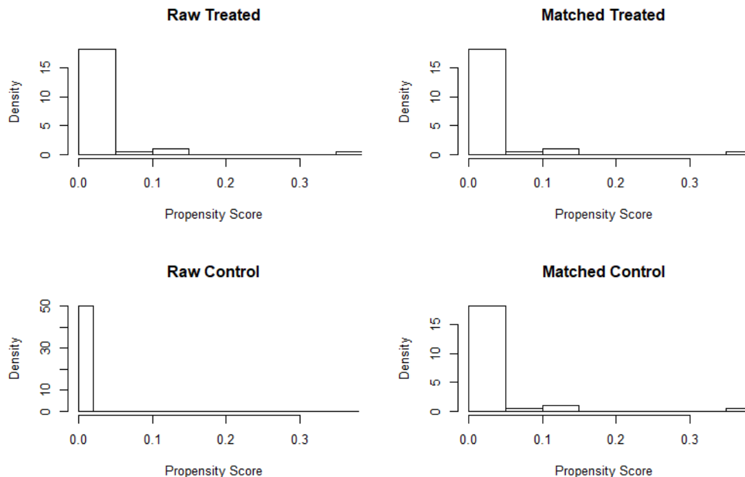
Gráfico 2. Histogramas de los índices de propensión correspondientes a la primera iteración del proceso de emparejamiento para el grupo de trabajadores/as por cuenta propia
