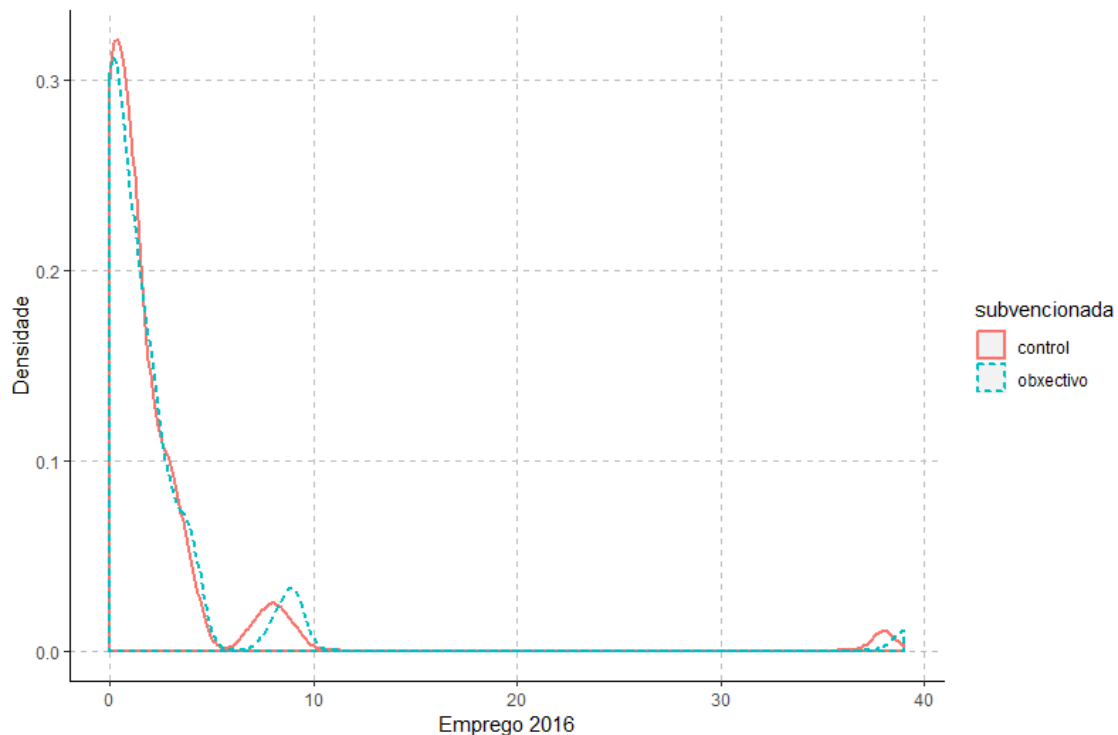
Gráfico 3. Funciones de densidad del empleo en 2016 de las empresas objetivo y control
