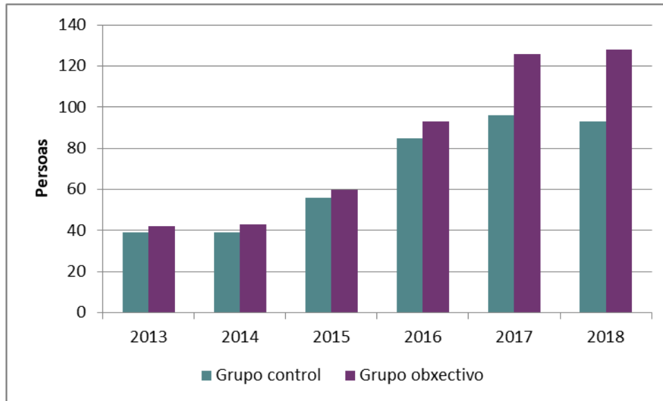
Gráfico 10. Comparativa de la evolución del empleo en Galicia de las empresas subvencionadas (grupo objetivo) y no subvencionadas (grupo control) para el grupo de sociedades/entes con personalidad jurídica
