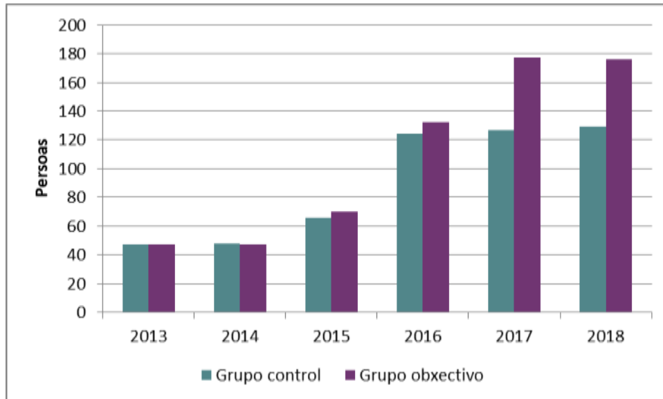
Gráfico 8. Comparativa de la supervivencia (empresas que continúan en activo en Galicia) de los grupos subvencionado (objetivo) y no subvencionado (control)
