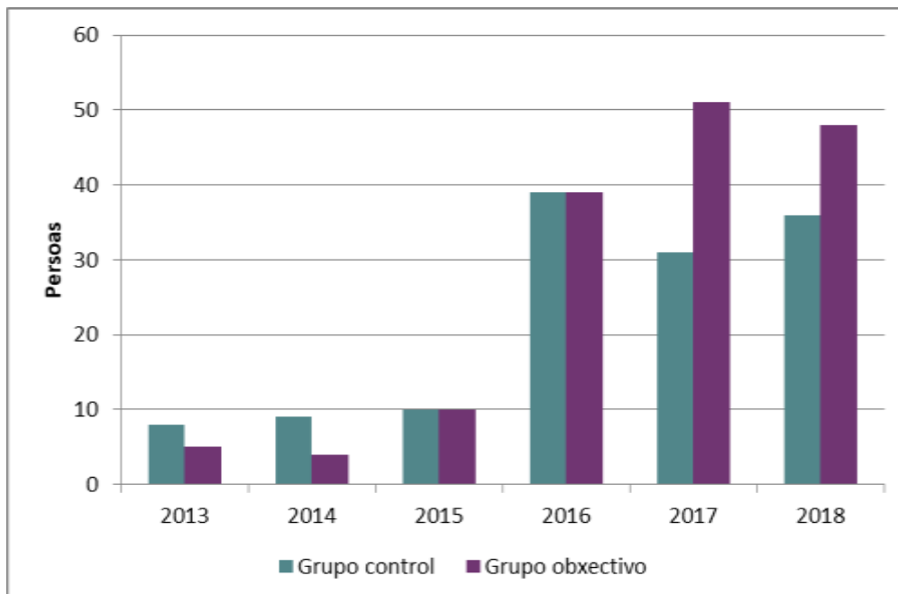
Gráfico 11. Comparativa de la evolución del empleo en Galicia de las empresas subvencionadas (grupo objetivo) y no subvencionadas (grupo control) para el grupo de trabajadores/as por cuenta propia
